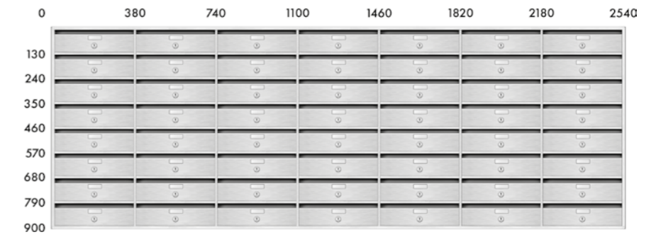
Profondità 250 mm.
